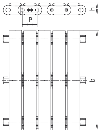
Varastolamelliketju 63 mm:n jaolla
