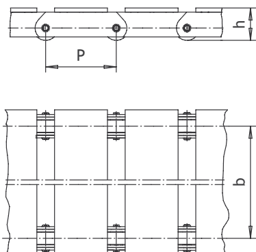
Varastolamelliketju 200 mm:n jaolla
