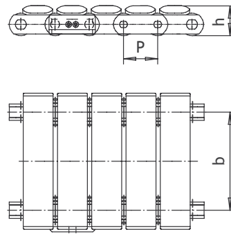
V-lamelliketju 63 mm:n jaolla
