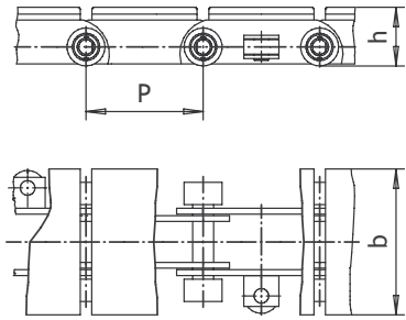
V-lamelliketju ulkopuolisin kulkurullin
